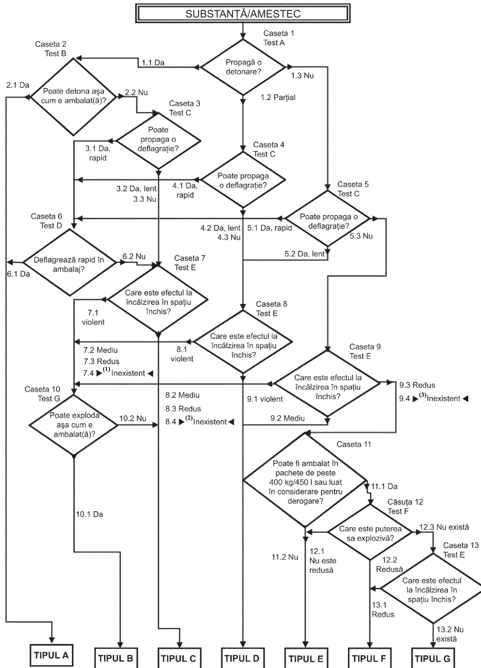
Figura 2.15.1 Peroxizi organici
